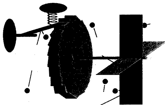
Abb. 1: Richard Feynmans Gedankenexperiment illustriert, warum sich aus einem Wärmebad im thermischen Gleichgewicht keine nutzbare Arbeit erzeugen lässt. Die Sperrklinke (links) ist nicht in der Lage, die Zufallsbewegung des Flügelrads (rechts) gleichzurichten, da sie selbst auch Kollisionen mit Gasteilchen ausgesetzt ist und eine Zufallsbewegung ausführt. Man könnte sich vorstellen, die Feder der Sperrklinke mit einem Maxwellschen Dämon zu ersetzen, der die Sperrklinke festhält, wenn das Flügelrad sich in die falsche Richtung dreht. Dazu müsste der Dämon aber Stöße von Gasteilchen absorbieren und würde bald selbst so viel Wärmebewegung ausführen, dass er zitternd aufgeben müsste.
