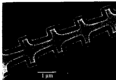
Abb. 4: Die Elektronenmikroskop-Aufnahme zeigt vier von insgesamt zehn Abschnitten einer Tunnelratsche für Elektronen. Die dunkleren Bereiche sind Gräben, die aus einer GaAs/AlGaAs-Heterostruktur geätzt wurden und so einen asymmetrischen Quantendraht definieren, der in Orange hervorgehoben ist. Jede der Verengungen stellt eine Energiebarriere für Elektronen dar. Das „Schaukeln“ des Ratschenpotentials wird mittels einer längs angelegten Wechselspannung erzeugt.
