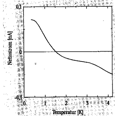
Abb. 5: Gemessener Nettostrom der in Abb. 4 gezeigten Elektronenratsche für eine angelegte Wechselspannung von 1 mV. Die Umkehr der Stromrichtung als Funktion der Temperatur ist charakteristisch für eine Quantenratsche.
